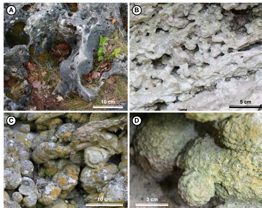
A – sommet du Rocher Carrosse, grès calcaire avec conduits de dissolution karstique (vue par audessus). B – base du rocher, sphérolithes centimétrique de calcite sableuse recimentée par des raies calcaires obliques. C – rocher "latéral" sphérolithes anastomosés et zonés au sein du sable non cimenté. D. sphérolithes avec rhomboèdres de calcite.
