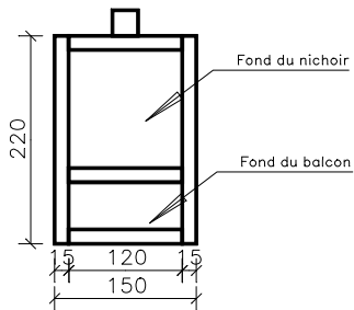
Vue de dessus (sans le toit)
