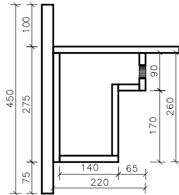
Vue de gauche (sans le coté)
